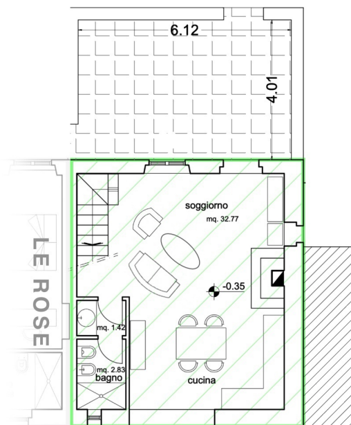
PIANTA PIANO TERRENO
